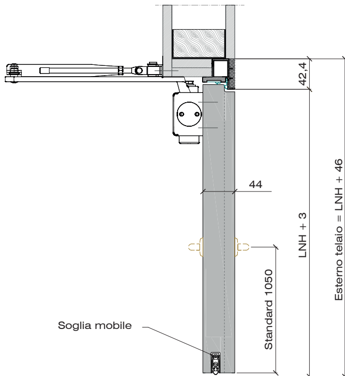
SEZIONE LONGITUDINALE
