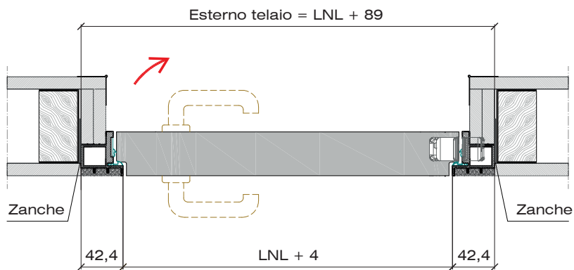
SEZIONE TRASVERSALE
